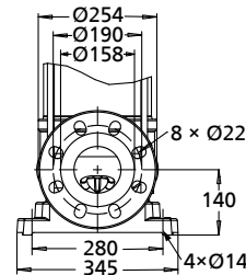
Fig. 63: Movitec VCF, PN 25/40
