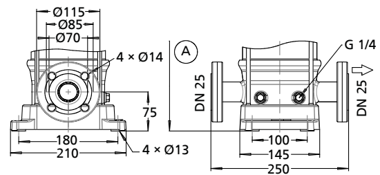
Fig. 13: Movitec VF, VSF
