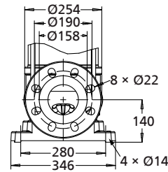
Fig. 61: Movitec VF/VSF, PN 25/40
