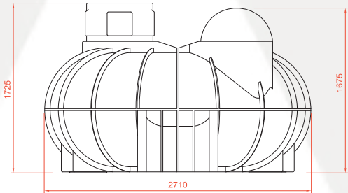
END ELEVATION
